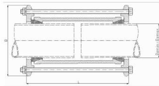
rys.2 korpus łącznika żeliwo
